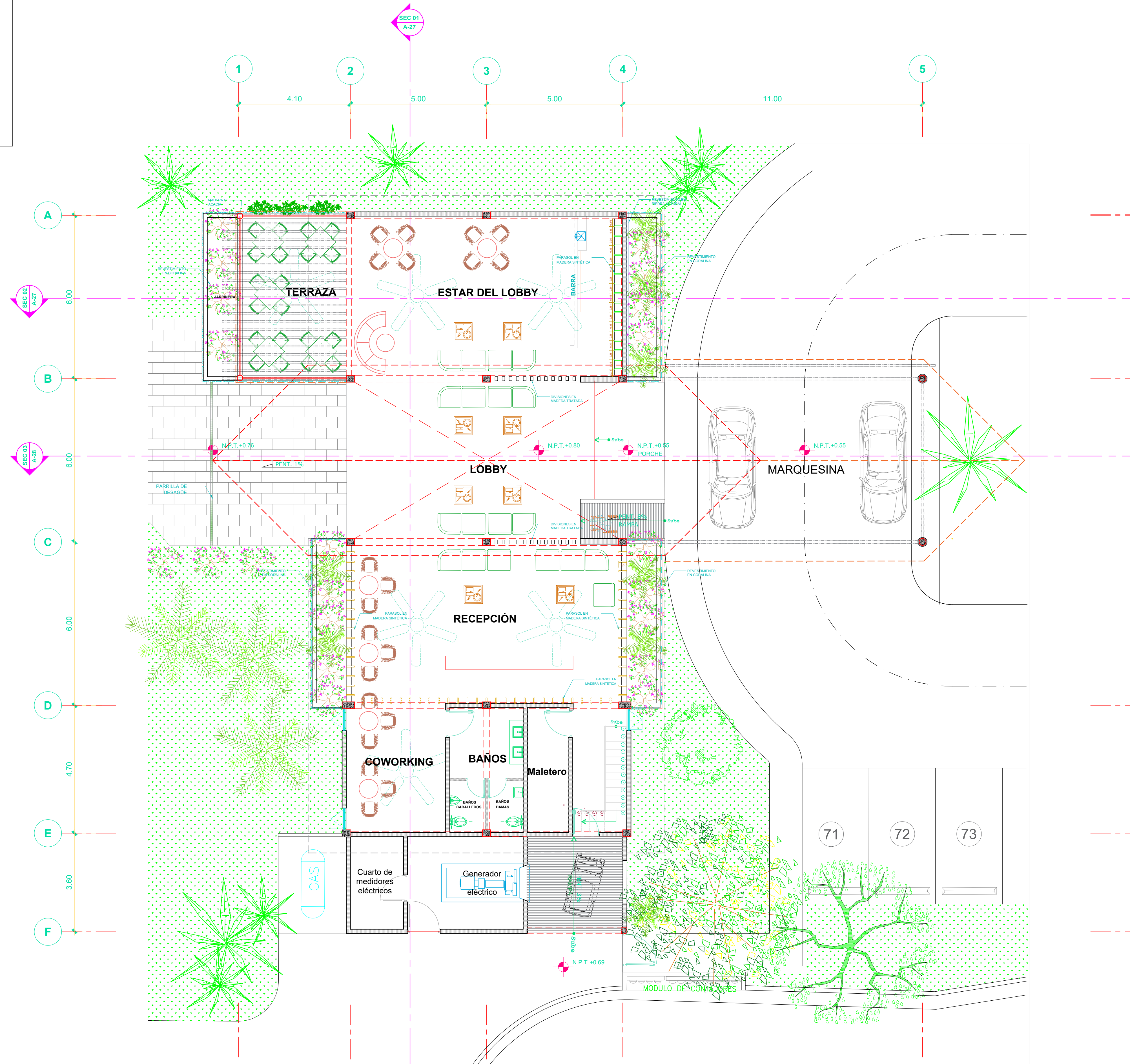
PLANTA ARQUITECTÓNICA 1er NIVEL Aparta- Hotel Galeras Bay Esc. 1:75 Edificio de Recepción
